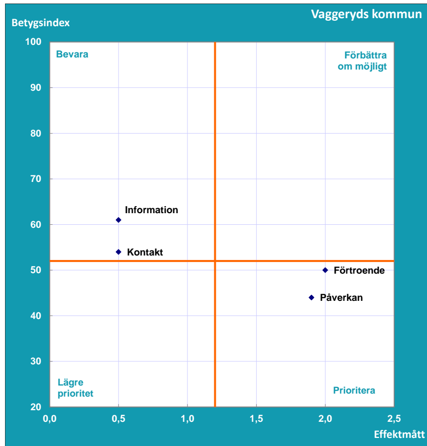
Diagram C1. Nöjd-Inflytande-Index (NII). Prioriteringsmatris för Vaggeryds kommun 2020.
