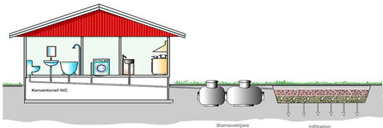
Bild: Principskiss för infiltration ( www.avloppsguiden.se )
